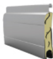
17 502 Lame 52 x 14mm Poids/m 2 : 5,1 kg/m 2 Largeur max. 4 ml
