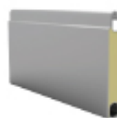
17 501 Lame 40 x 8mm Poids/m 2 : 2,9 kg/m 2 Largeur max. 2,5 ml
