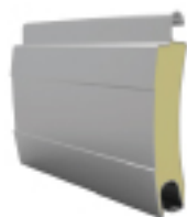
17 503 Lame 55 x 14mm Poids/m 2 : 3,6 kg/m 2 Largeur max. 3,5 ml
